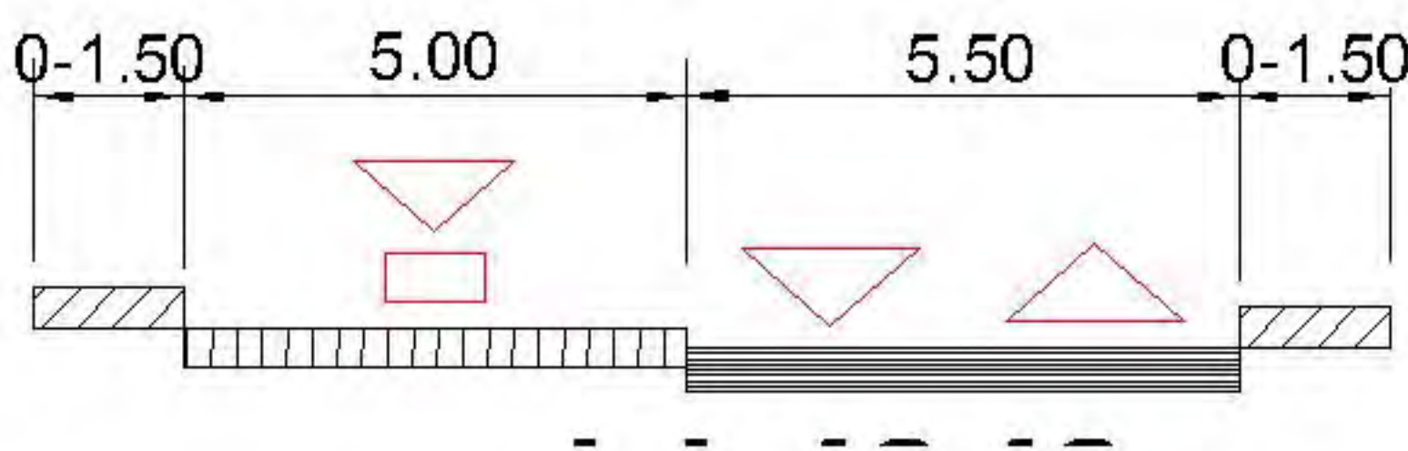
presjek 15-15
